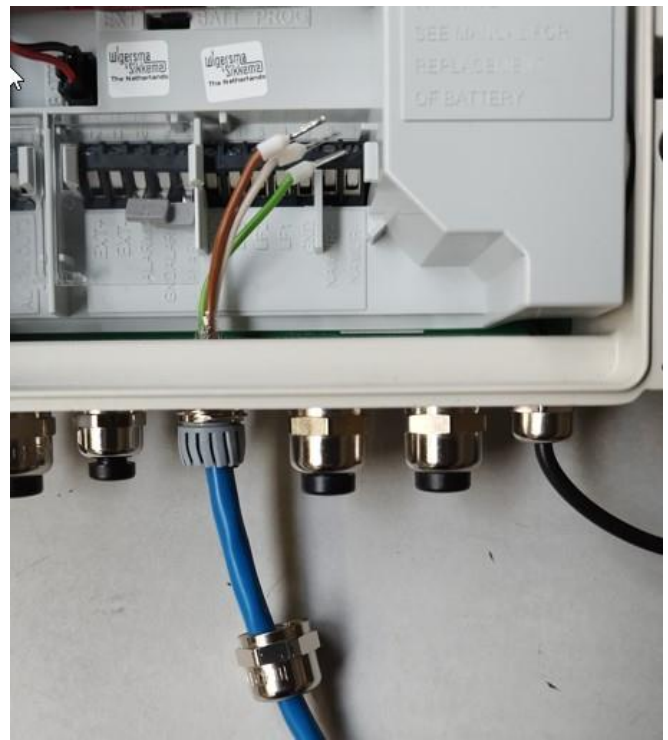
8: Druk de afdichthuls in de kabeldoorvoerwartel en draai deze enigszins vast.
