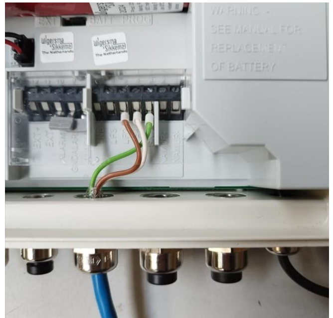
10: Plaats de transparante afdekkap
